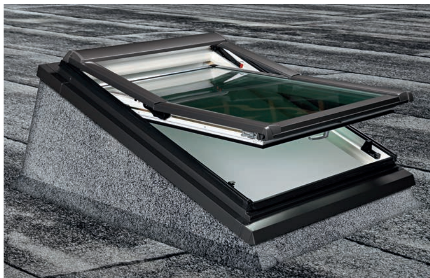
Sklon okna v zdvihovom ráme je zvýšený o bezpečných 20° proti zatekaniu.
