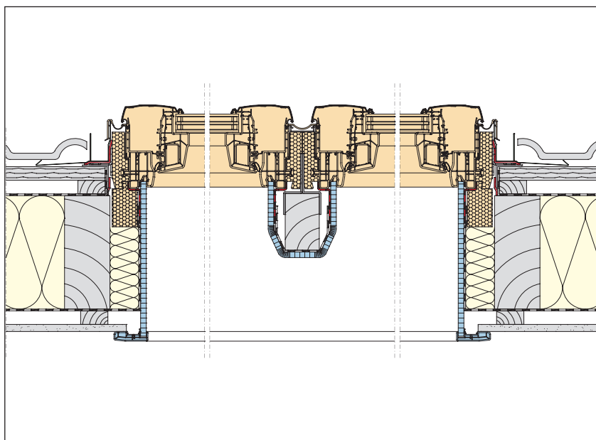
Rez zostavu dvojice strešných okien bez stredovej krokvy
