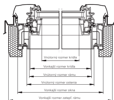
rez B-B
