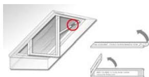
Kyvné a výsuvno-kyvné okno R4/R7
