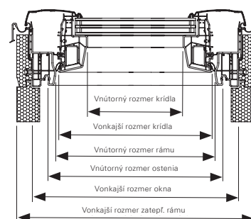
rez B-B
