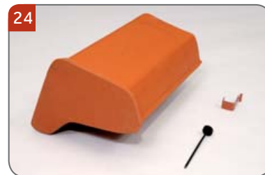
Univerzální pultový hřebenáč zakončovací, levý s jednou příchýtkou hřebenáče HO + N a s jedním vrutem Pro napojení pultové hrany na štítovou.
