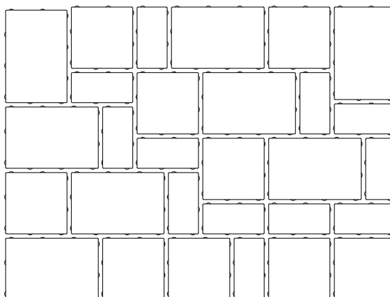
Obr. č. 17 Kombi 6, Kombi 8 - rozložení formátů na paletě (viz kladecí plán č. 6)
