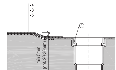
3.2.b Detail - Verbindungsfolie aus Bitumenstreifen
